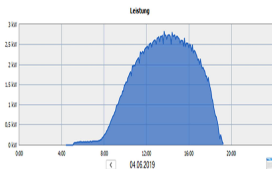
Tagesertrag 4.6..2019
