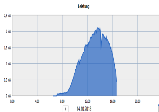
Tagesertrag 14.10.2018
